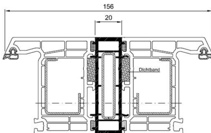
Obr. 42b. Příklad spojení oken z PVC profilů
