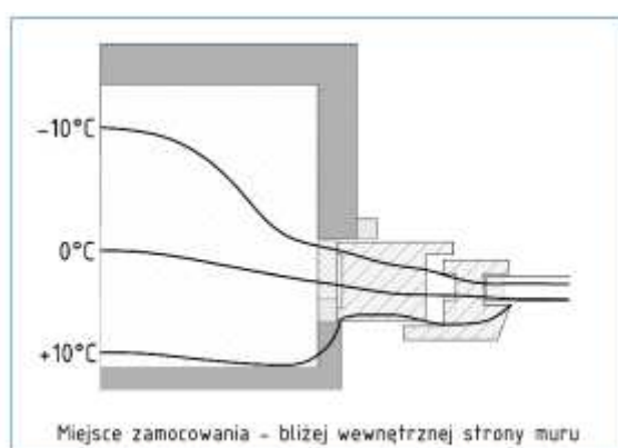
Fig. 5b Emplacement de fixation – plus près du côté intérieur du mur
