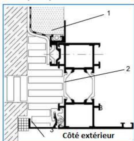
Fig. 24. Exemple d'étanchéité de l'espace entre une fenêtre en aluminium et le dormant sans jambage dans un mur à ossature.
