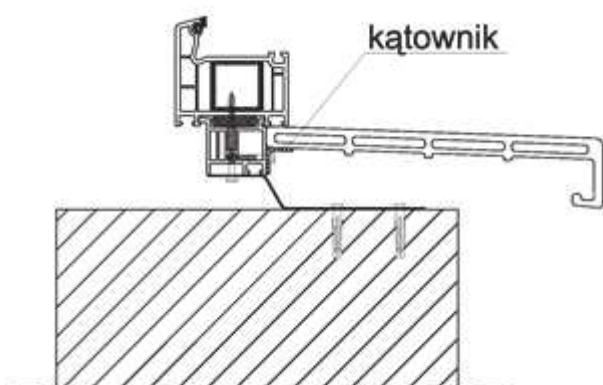
Fig. 40. Illustrant la méthode de fixation supplémentaire du seuil par l'utilisation d'un cornière vissée à la moulure de seuil.
