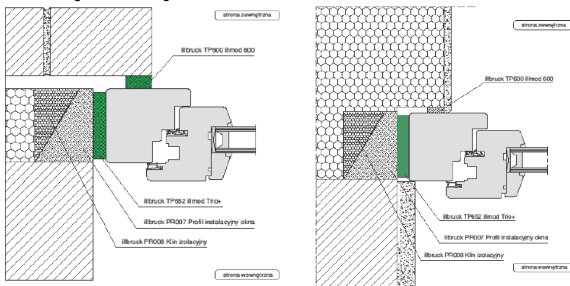
Fig. 11a. Montage de la fenêtre dans la couche d'isolation.
