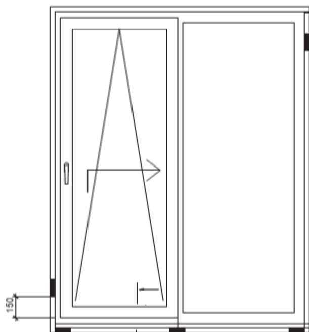
Fig. 9. Disposition des cales de support et des cales d'écartement dans une coulissante PSK.
