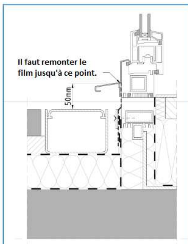
Schéma n° 31 Exemple d'étanchéité du seuil des portes-fenêtres avec évacuation de l'eau de pluie.
