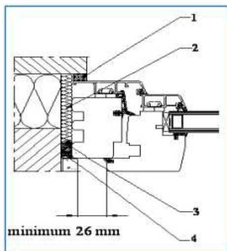
Fig. 23. Exemple d'étanchéité de l'espace entre une fenêtre bois-aluminium et le dormant
