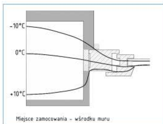
Fig. 5c Courbes des isothermes en fonction du positionnement de la fenêtre.
