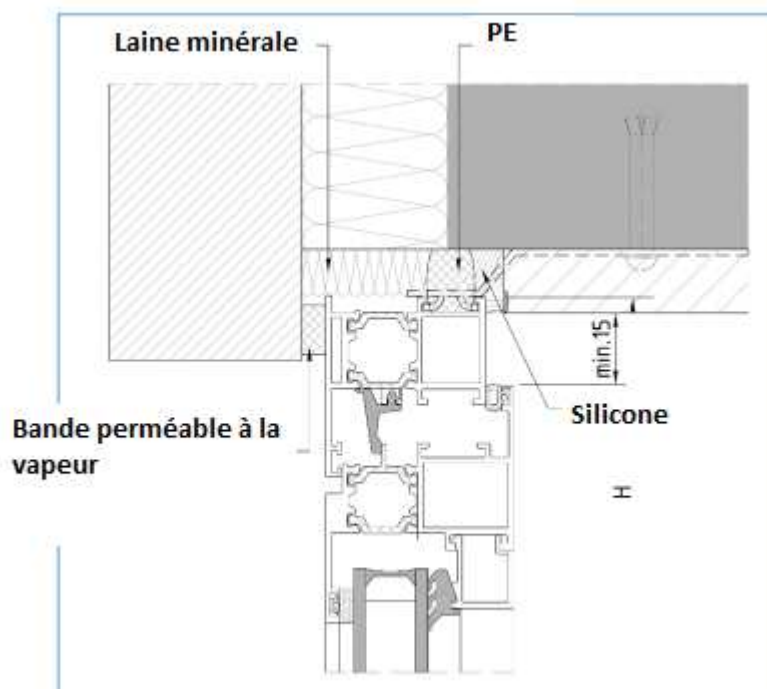
Fig. 28. Exemple d'étanchéité du joint du linteau d'une fenêtre en profilés aluminium.
