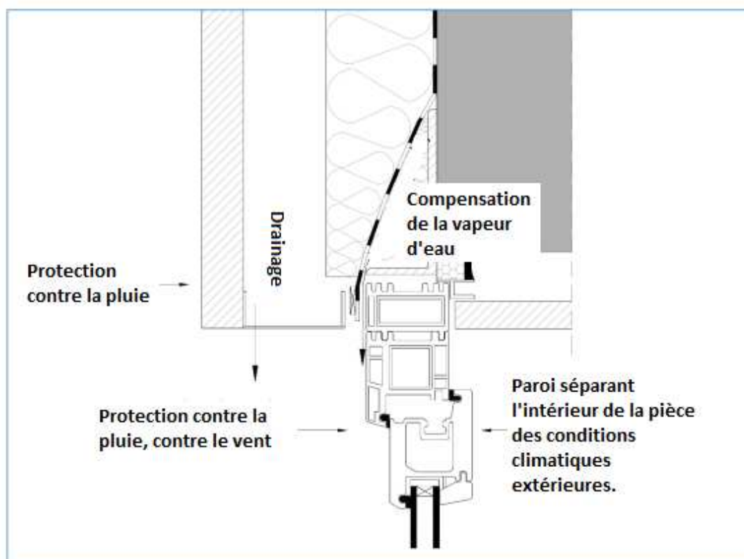
Fig. 26 Exemple d'étanchéité du joint du linteau.
