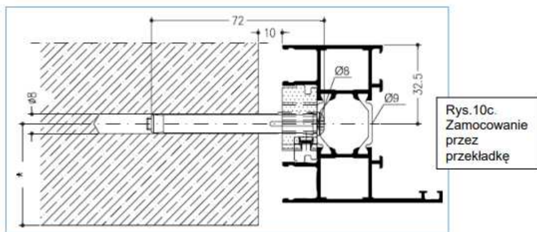
Fig. 10c. Fixation par entretoise
