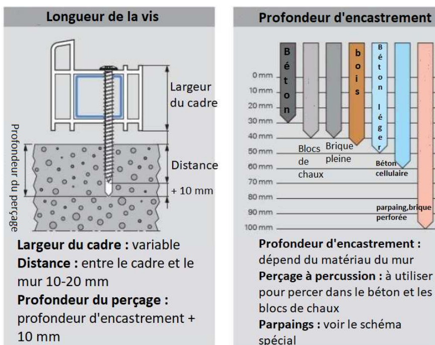
Fig. 10f. Règles de fixation des vis dans différents matériaux
