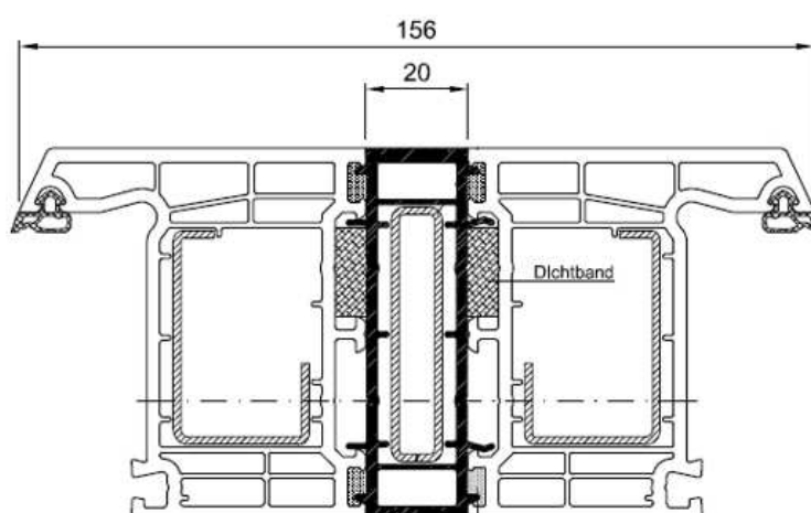
Fig. 42b. Exemple de l'assemblage des fenêtres en profilés PVC
