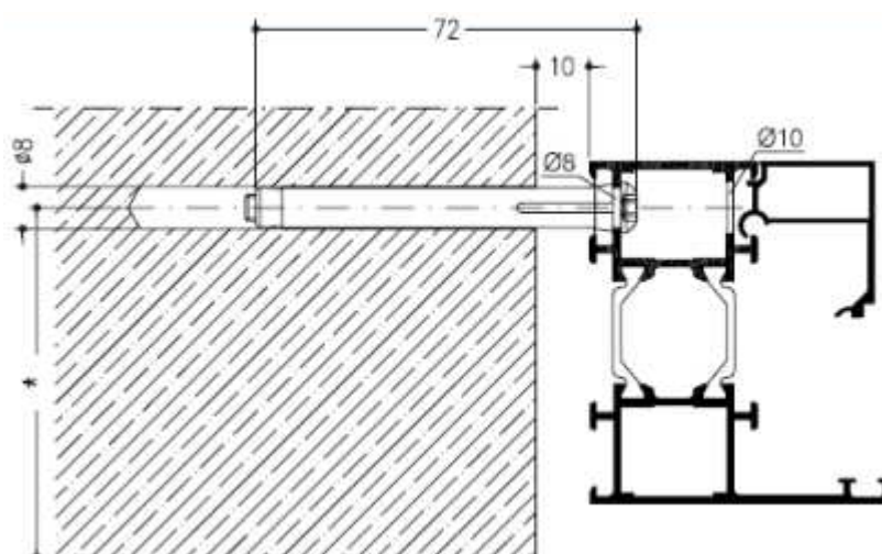
Fig. 10e. Fixation par profil en aluminium
