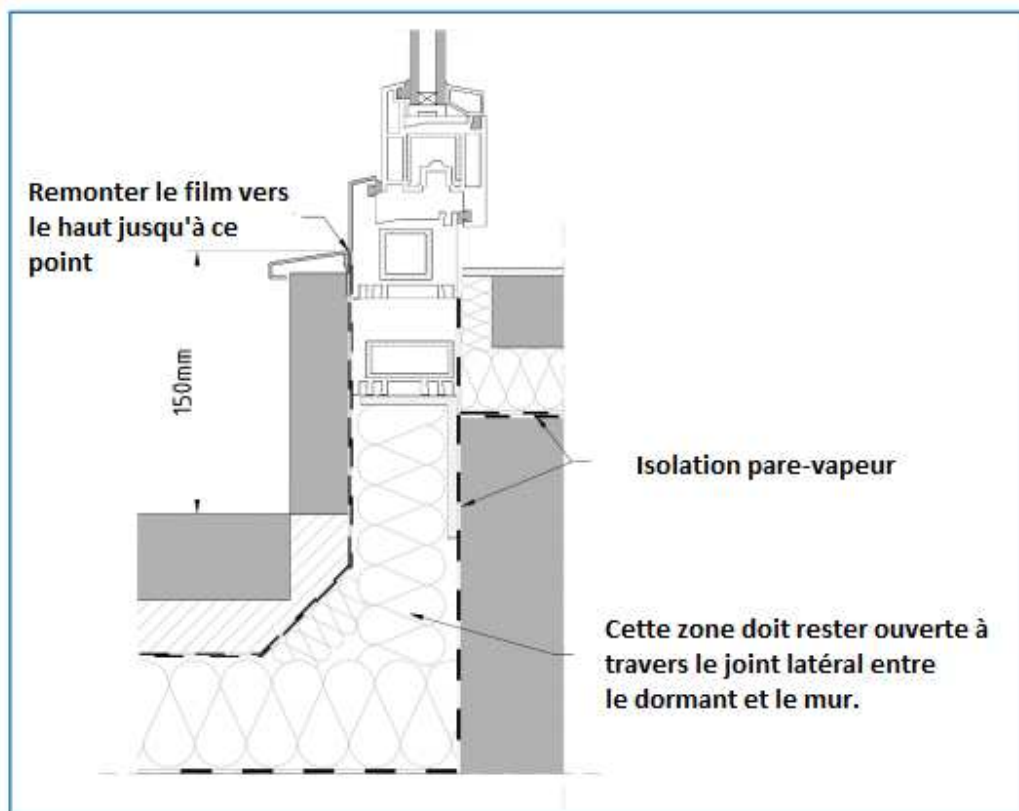
Fig. n° 29. Exemple d'étanchéité du seuil des fenêtres/portes-fenêtres coulissantes.
