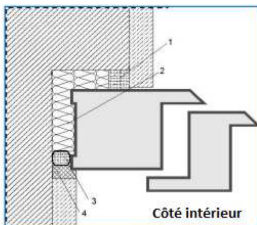
Fig. 22. Étanchéité de l'espace entre la fenêtre et le dormant dans un mur plein avec jambage
