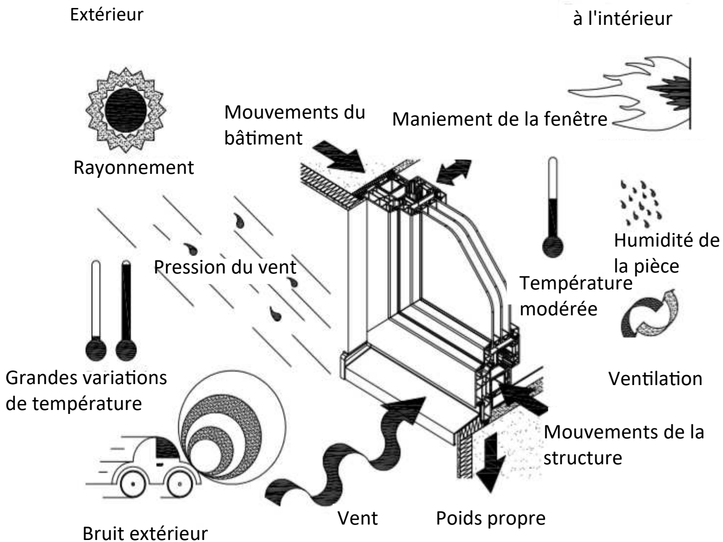
Fig. n° 1 : Fonctions de la fenêtre
