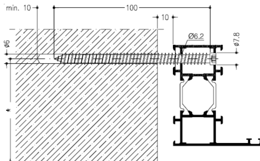
Fig. 10c. Fixation par entretoise
