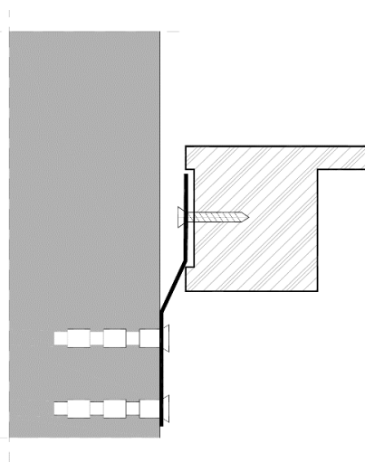
Fig. 10d Fixation avec l'utilisation d'un ancrage
