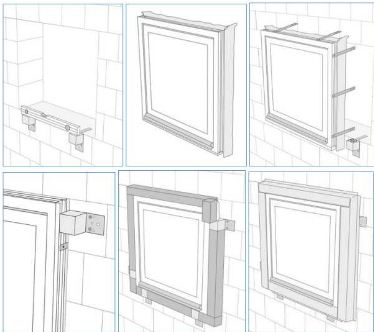
Fig. 11b. Phases de montage de la fenêtre dans la couche d'isolation
