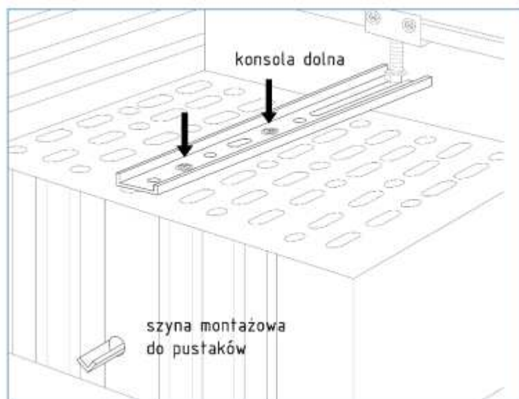
Fig. 13 Exemple de fixation de la console inférieure au mur en parpaings
