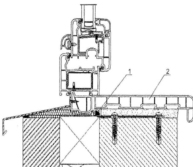
Fig. 41. Exemple de fixation de l'appui de fenêtre intérieur à une fenêtre en PVC.
