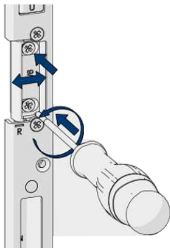
Fig. 93 Autre perspective de réglage de la charnière
