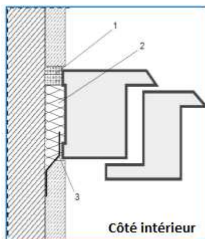
Fig. 21. Étanchéité de l'espace entre la fenêtre sans jambage et le dormant
