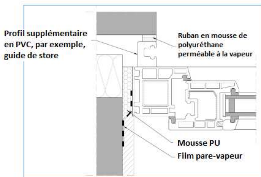
Fig. 26 Exemple d'étanchéité du joint du linteau.
