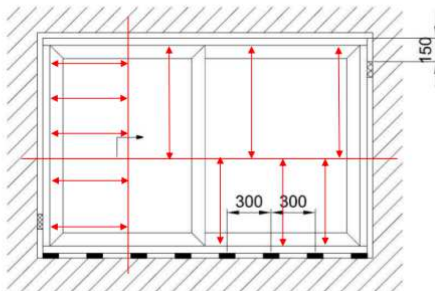
Fig. 10. Disposition des cales de support et des cales de distance dans le coulisant HST
