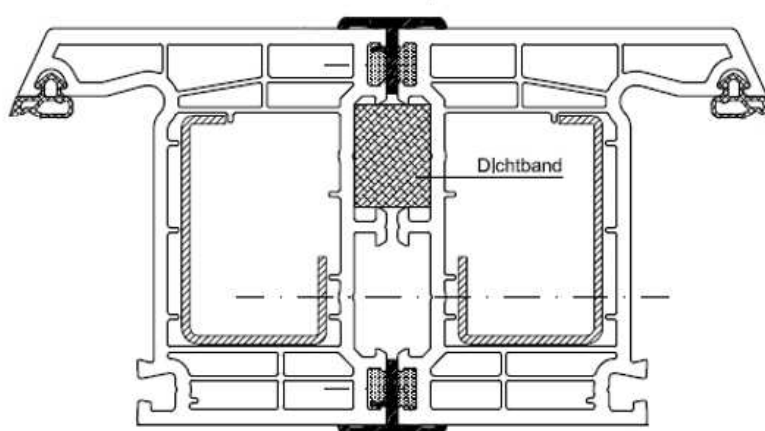
Fig. 42a. Exemple de l'assemblage des fenêtres en profilés PVC.
