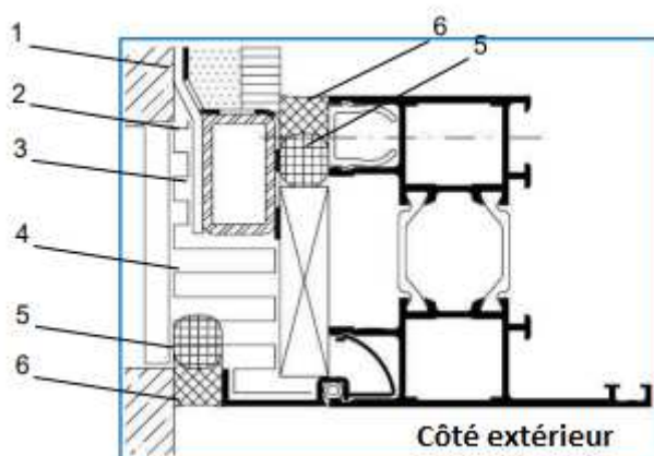
Fig. 25. Exemple d'étanchéité du joint entre une fenêtre en aluminium et l'ébrasement.
