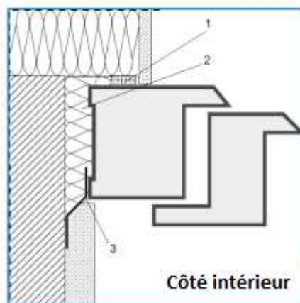
Fig. 20 Étanchéité de l'espace entre la fenêtre et le dormant dans un mur avec isolation extérieure
